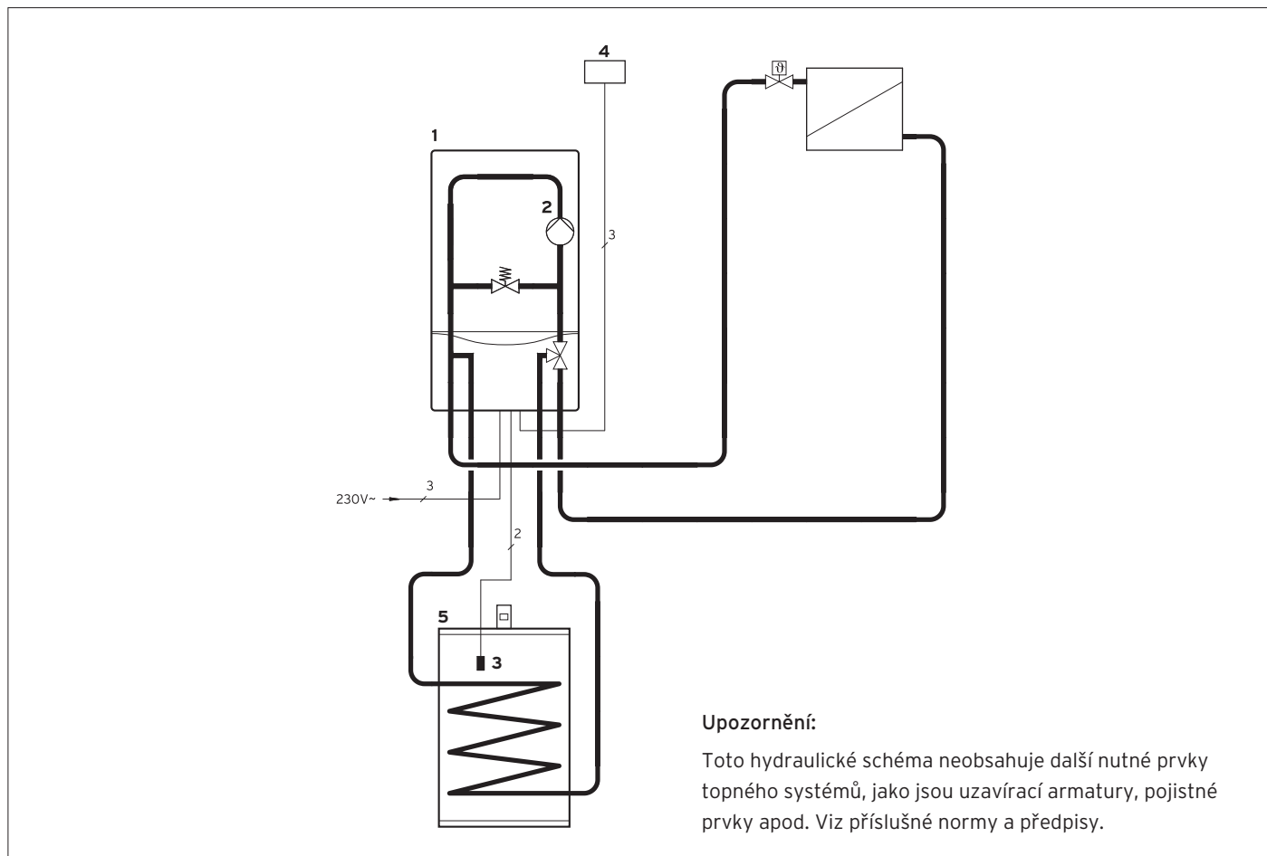
Příklad 1: jednokruhový topný systém s přípravou teplé vody
