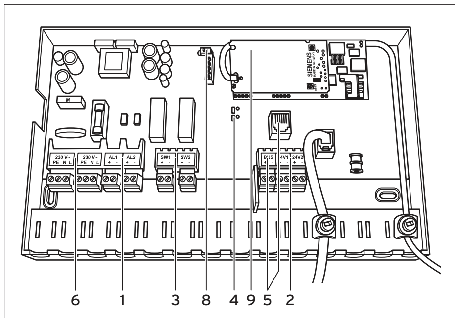
Připojení vrnetDIALOG 860/2
