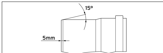
10.6 Zkosení trubky
