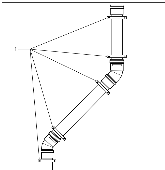
12.7 Příklad upevnění vedení spalin s kolenem 45°
