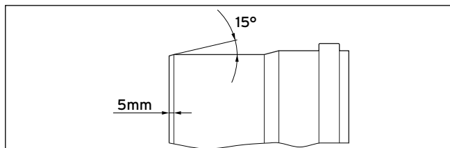
13.5 Zkosení trubky
