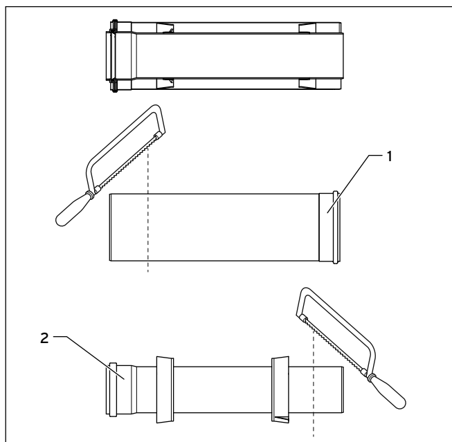
10.15 Zkrácení prodloužení
