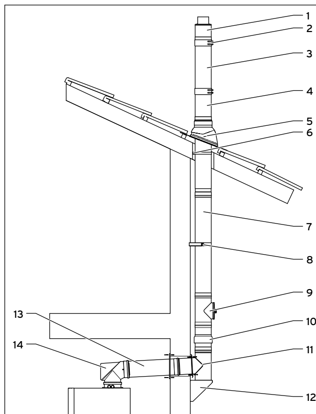
10.1 Schéma systému vedení spalín
