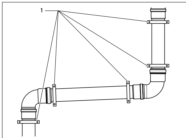
12.6 Příklad upevnění vedení spalin s kolenem 87°
