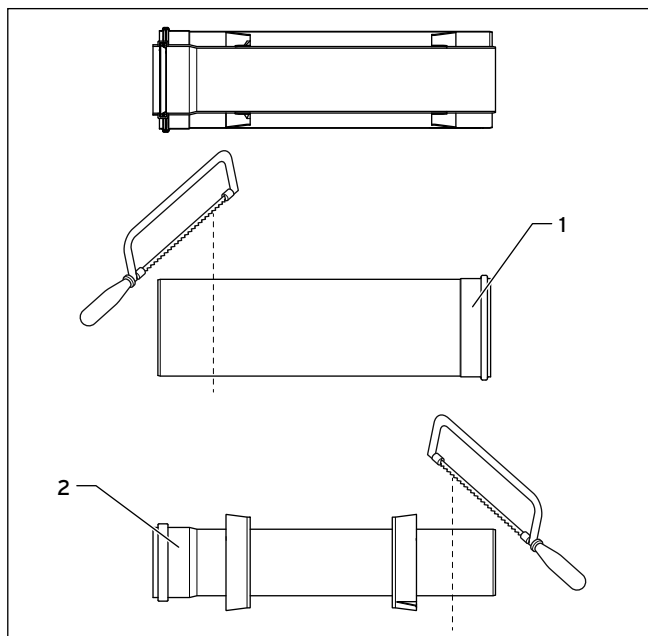
13.4 Zkrácení prodloužení
