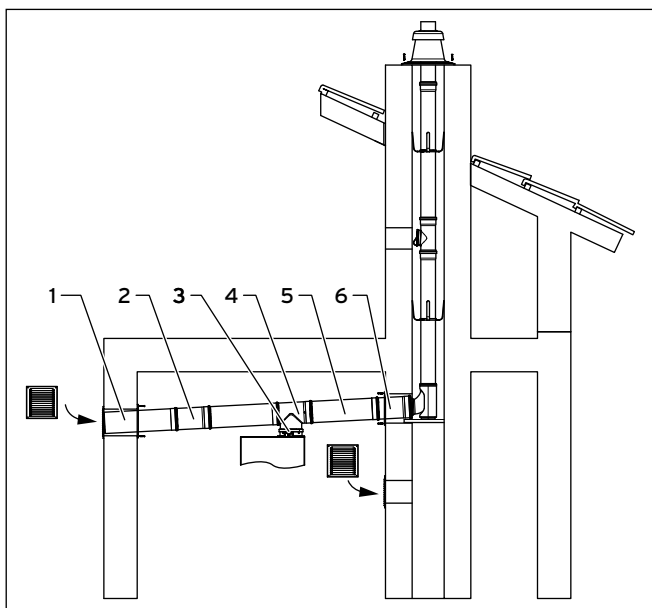
9.5 Přívod vzduchu vnější stěnou
