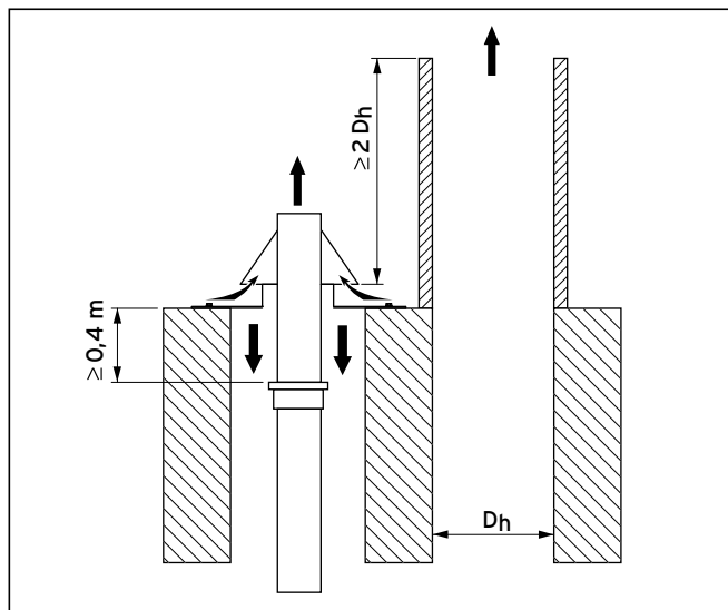
8.3 Výška kouřovodu nad vedením spalin z PP s vyústěním z nerez - systém nezávislý na vzduchu z místnosti
