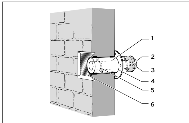
9.4 Montáž dílu pro přívod vzduchu
