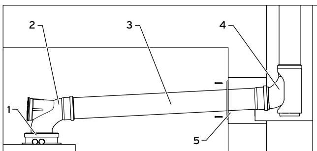
12.5 Montáž vodorovného vedení spalin
