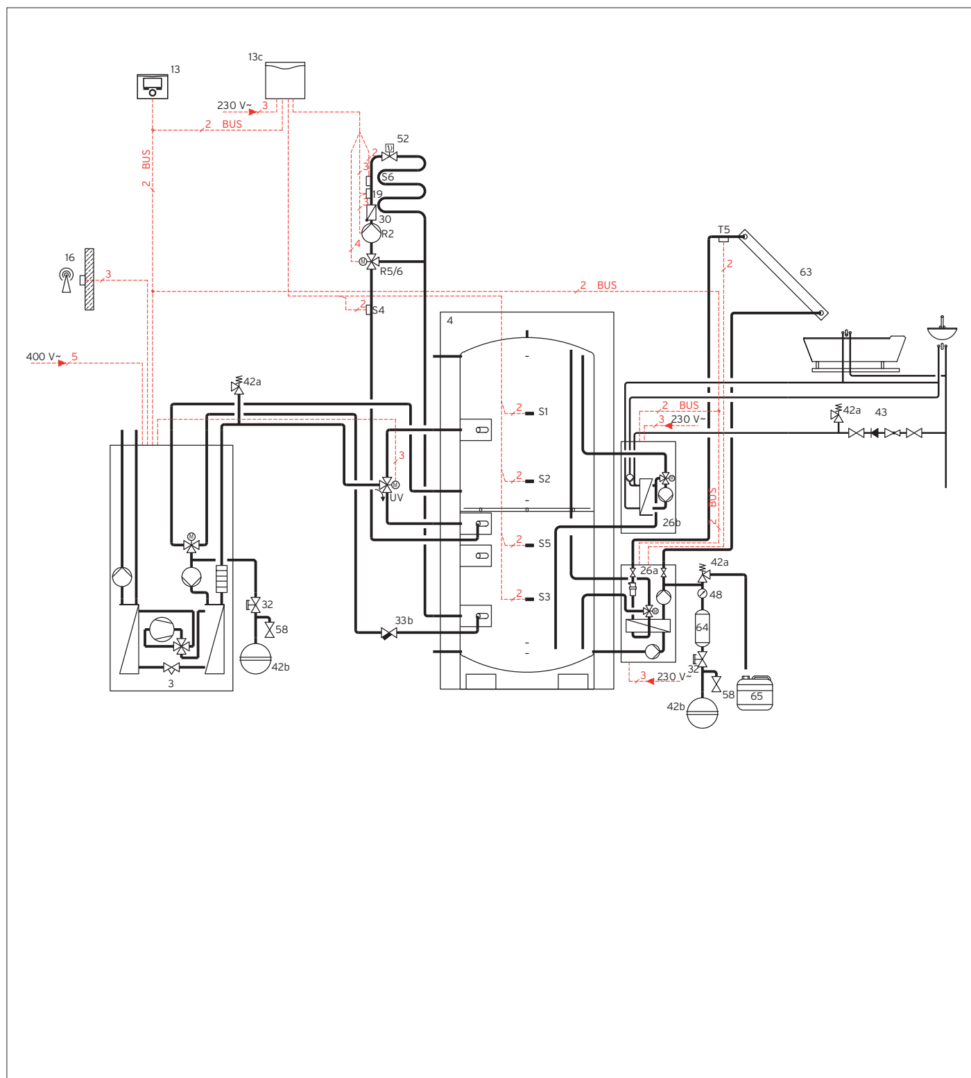
Hydraulické schéma
