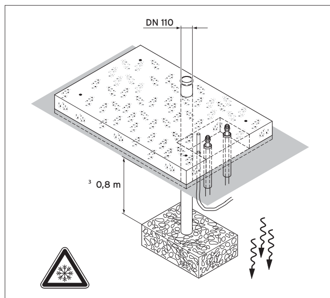
Připojení do betonového základu
