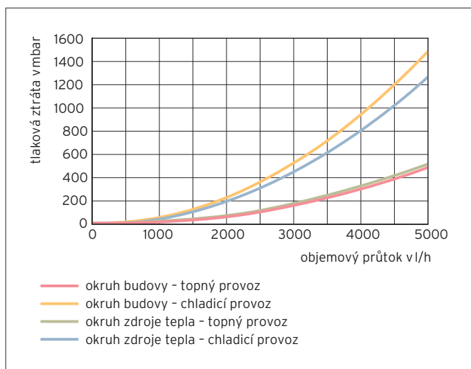
Graf tlakové ztráty VWZ NC 19 /4
