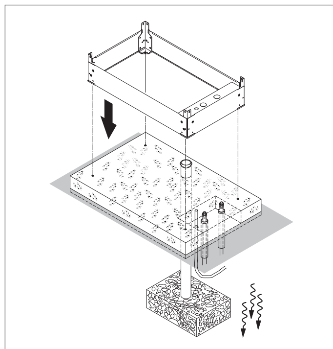
Montáž soklu
