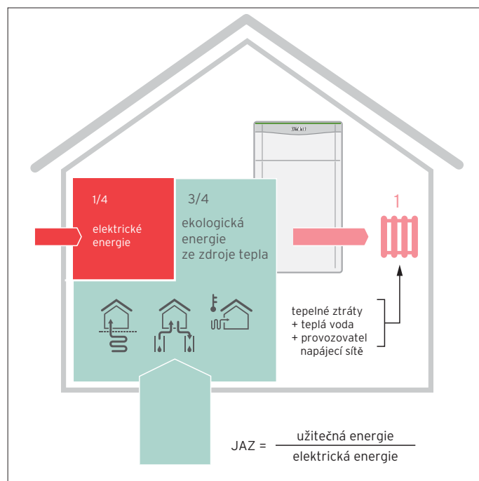
Roční pracovní faktor a dimenzování zdroje tepla
