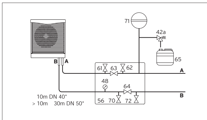
Armatury v okruhu s nemrznoucí směsí
