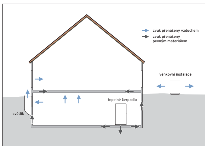
Cesty přenosu zvuku v budově
